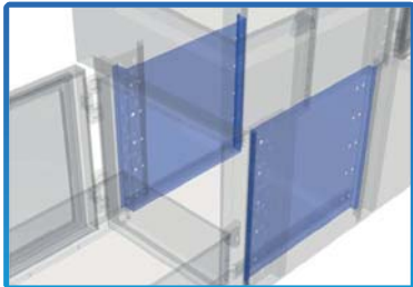
Schubladenbefestigungsbleche zur Aufnahme der Schubladen * (Links und rechts verwendbar)
